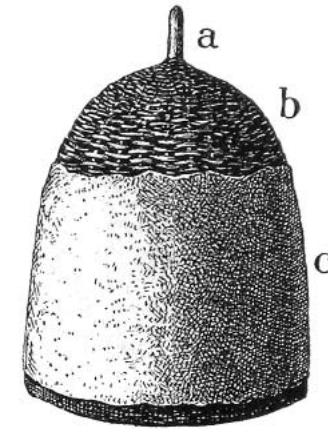
Glockenstülper aus Korbweide [Rutenstülper]. a, Tragegriff; b, kleines Holz; c, Putzschicht aus Pourget (Gemisch aus Ton und Kuhdung)
