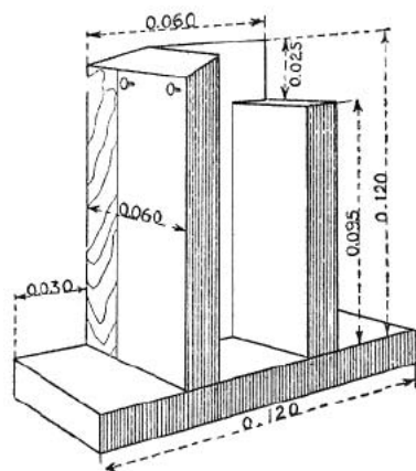
Hölzerner Beutenfuß, den man mit vier Drahtstiften an jeder Ecke des Bodenbrettes befestigt.
