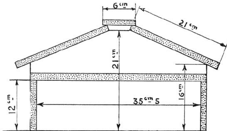
Schnittbild des Hüttendachs.
