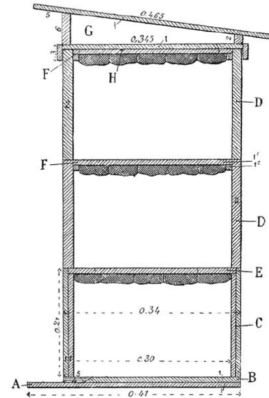
Schnittbild der Volksbeute.
