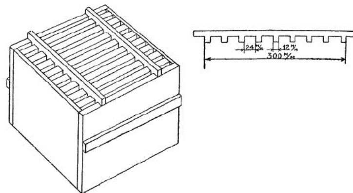
LEHRE, um die Wabenträger zu platzieren und sie während des Annagelns zu halten.
