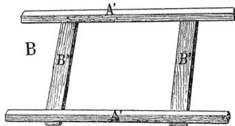
Leistenuntersatz für die Zargen.
